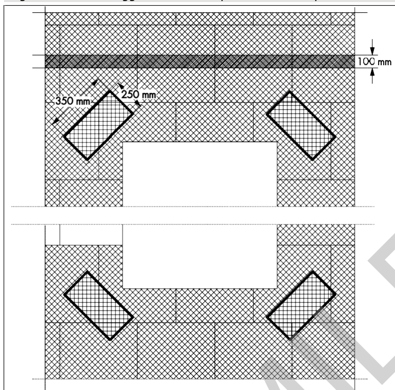
Figura 7 Armatura aggiuntiva in corrispondenza delle aperture
