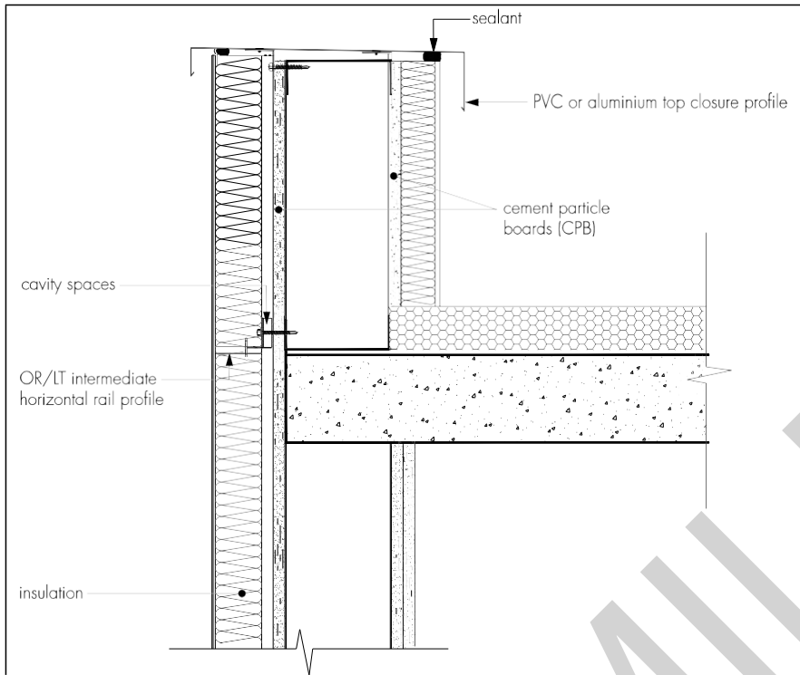
Figura 8 Disegno tipico parapetto del tetto - Particolare
