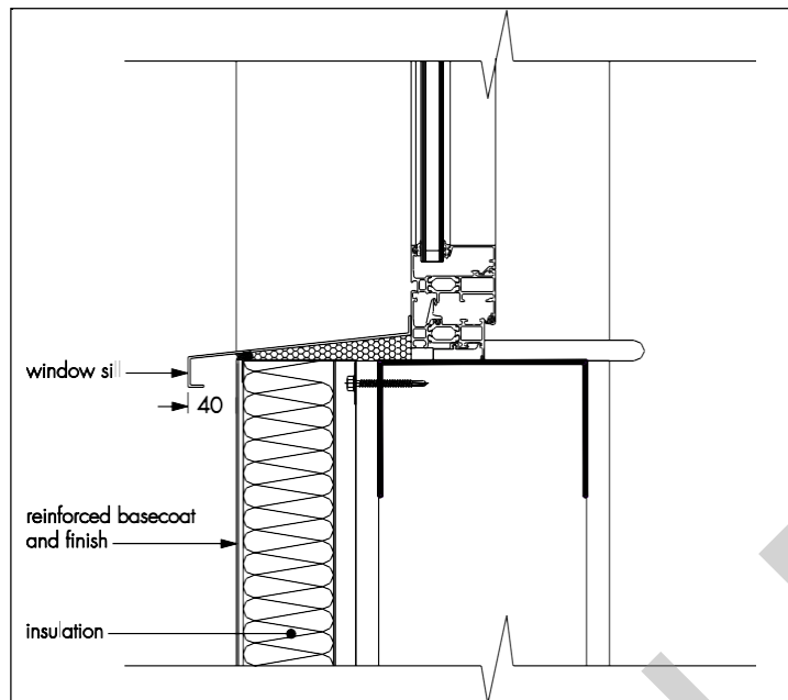
Figura 10 Davanzale finestra - Particolare
