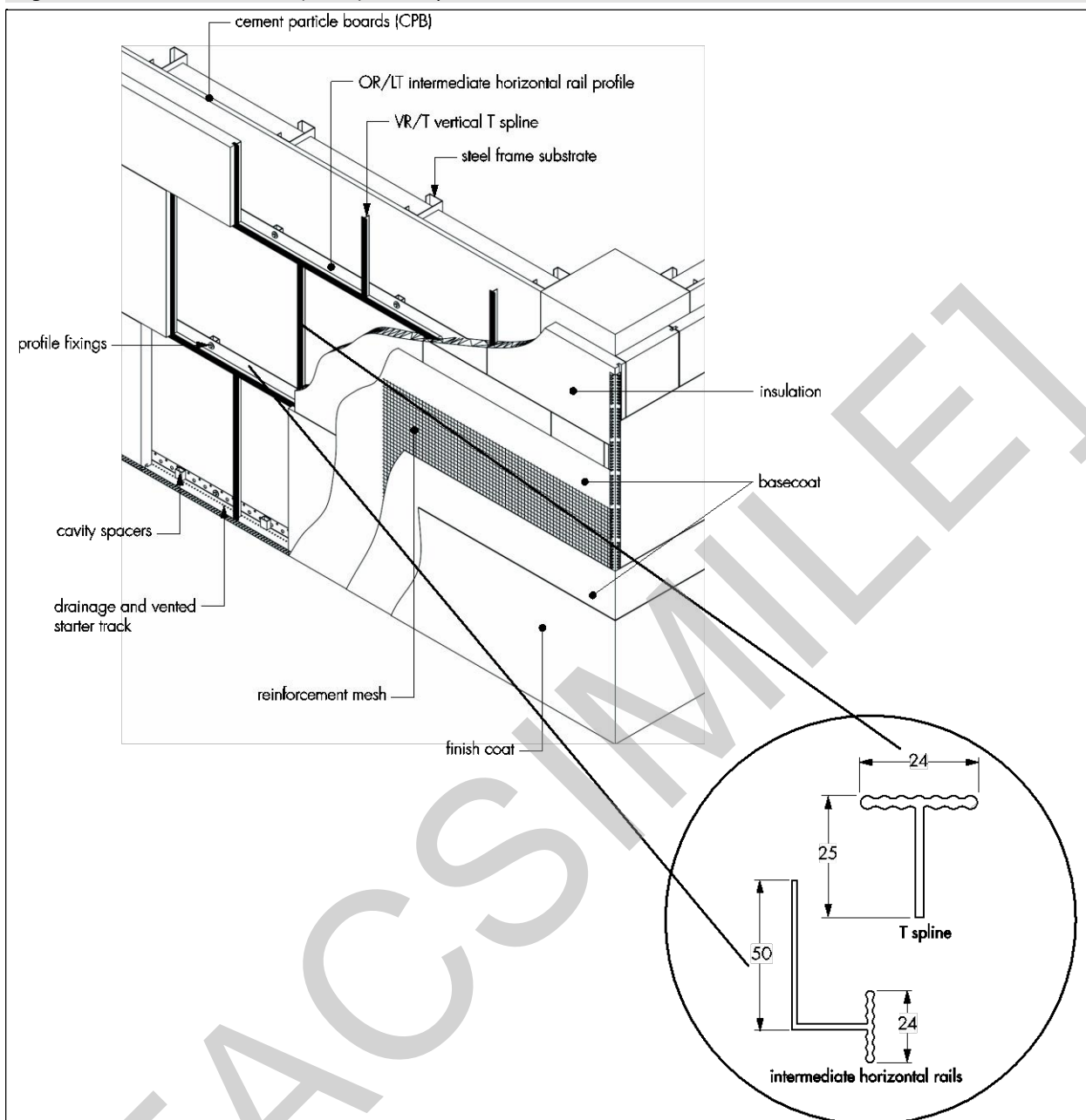
Figura 1 Termok8 Meccanico (LWSF) — componenti del sistema di isolamento termico esterno
