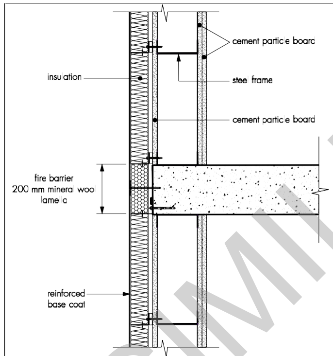
Figura 2 Barriera tagliafuoco
