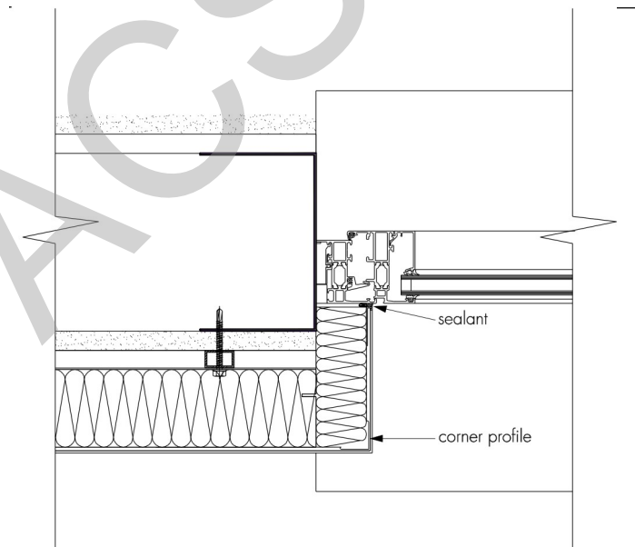
Figura 9 Disegno tipico apertura - Particolari
